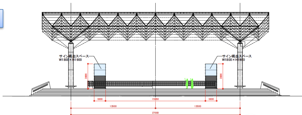
立面図
